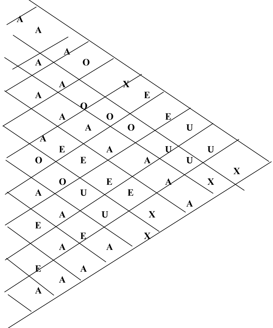
Рис. 3.2. Сітка мазера
